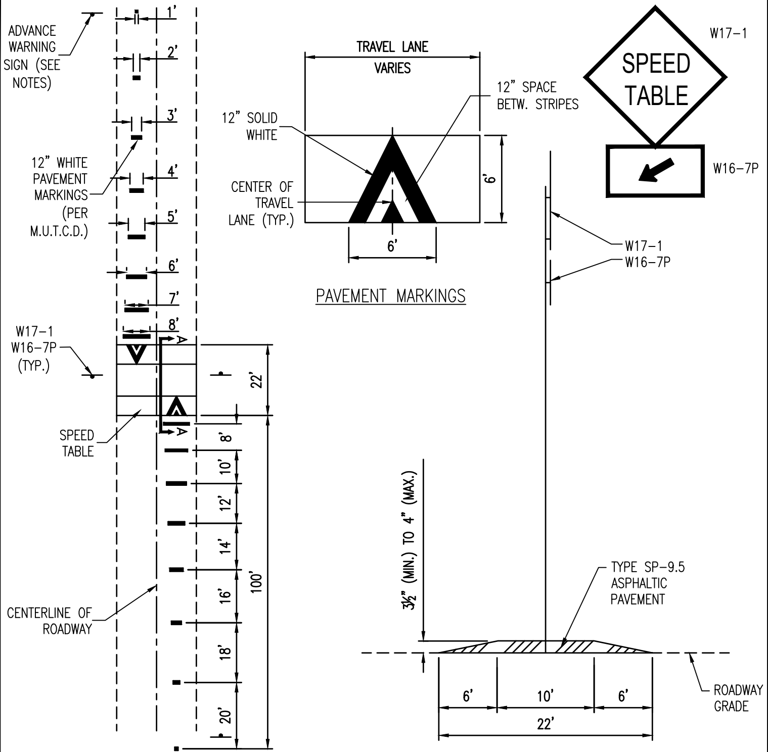
PLAN N.T.S.
