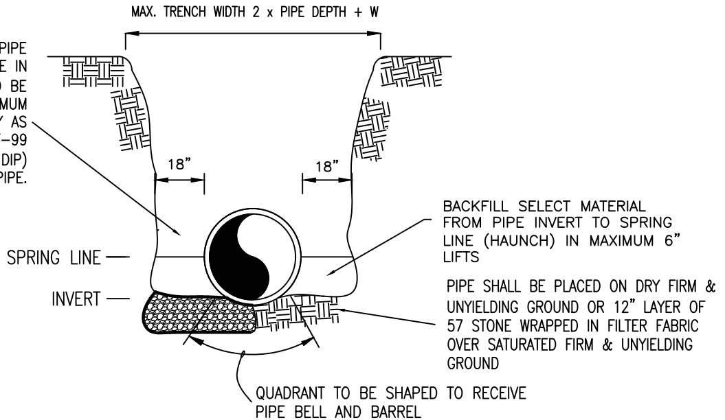
TRENCH DETAIL N.T.S.
