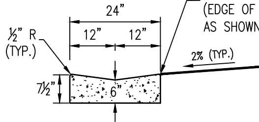
VALLEY GUTTER N.T.S.
